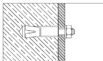
Vorsteckmontage (Innengewindeanker)
